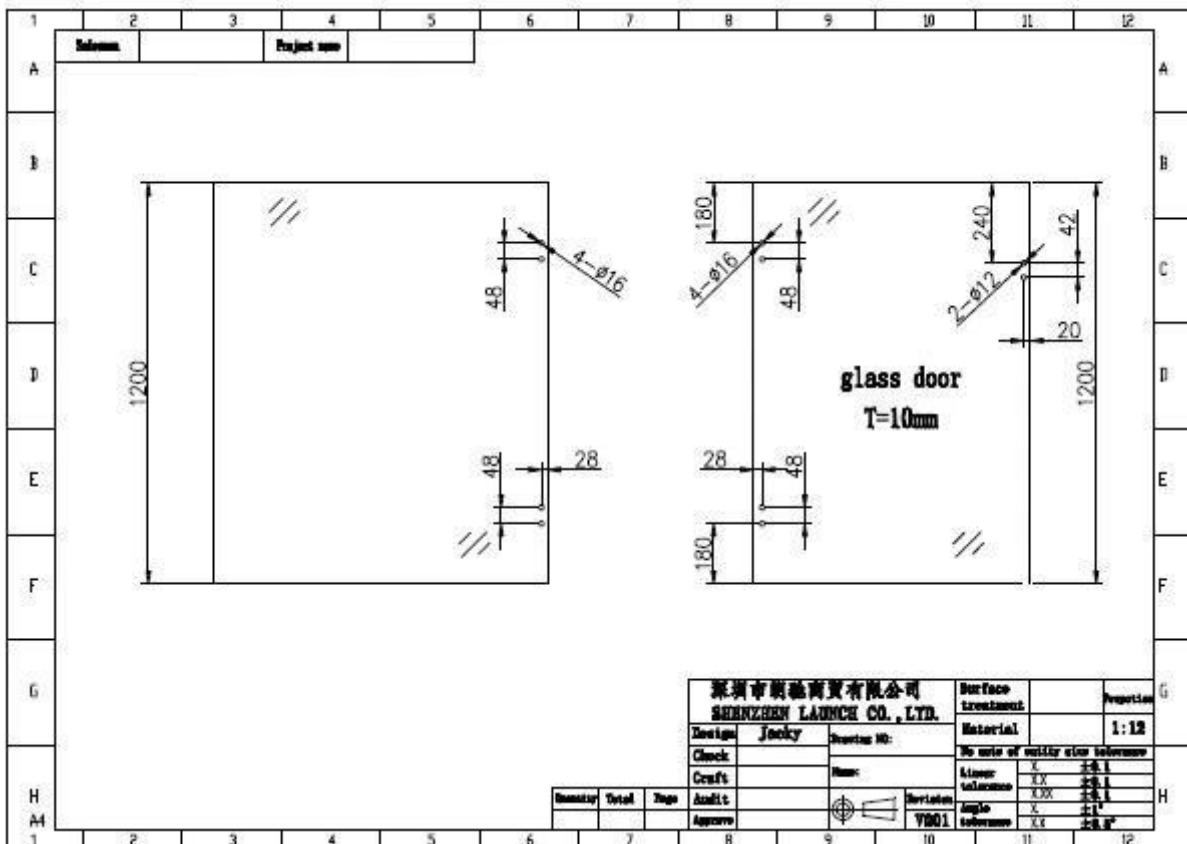
Glastürscharnier Standard Glaspaneel Löcher Position Zeichnung
