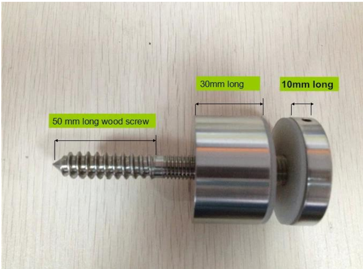
Standoff barandilla de vidrio
