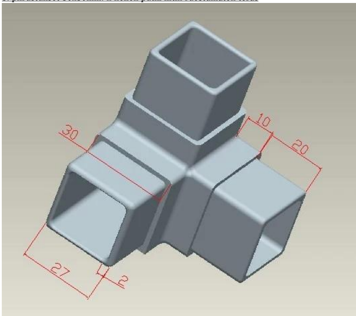
3. piirustukset 30x30mm: n neliön putki liitin ruostumaton teräs
