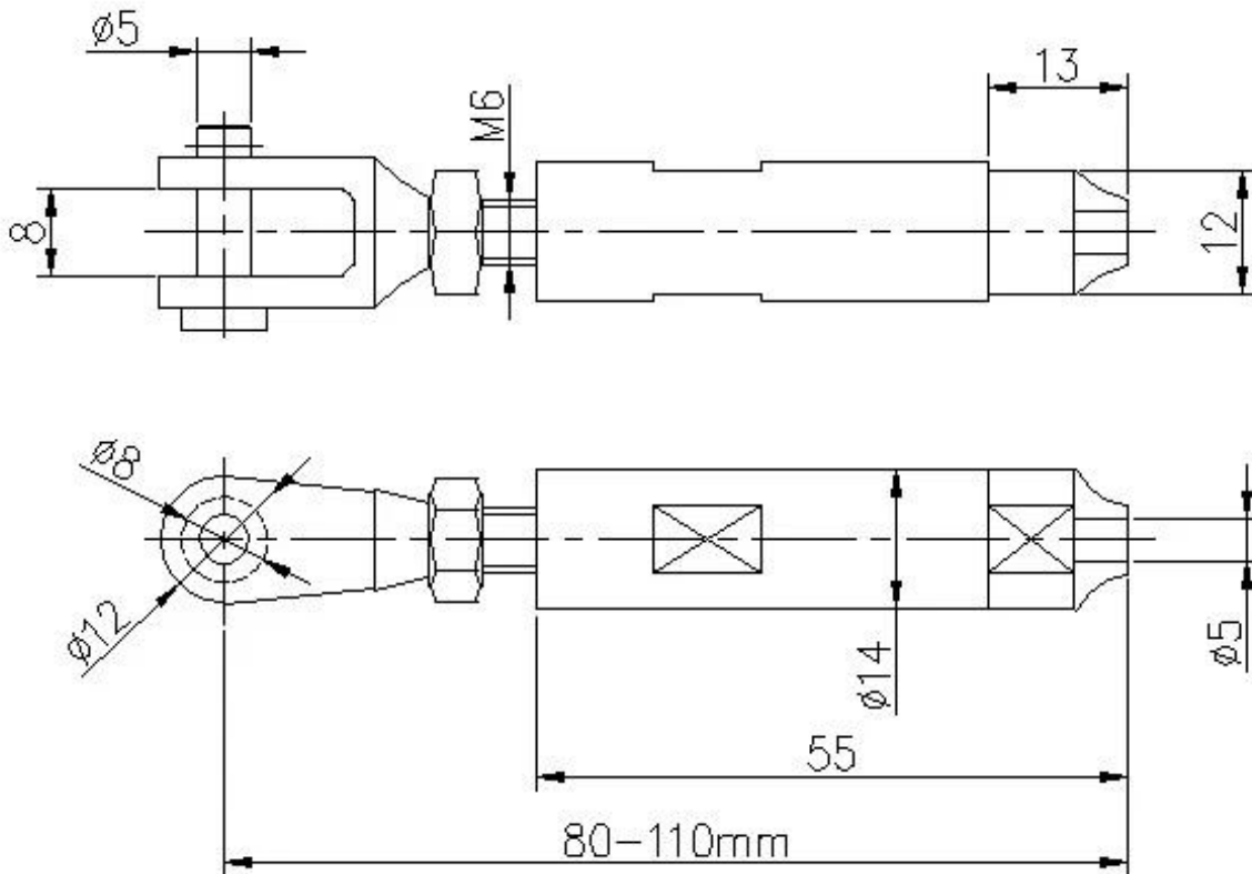
Valmistuskuvat teräsköyden kiristimestä T803
