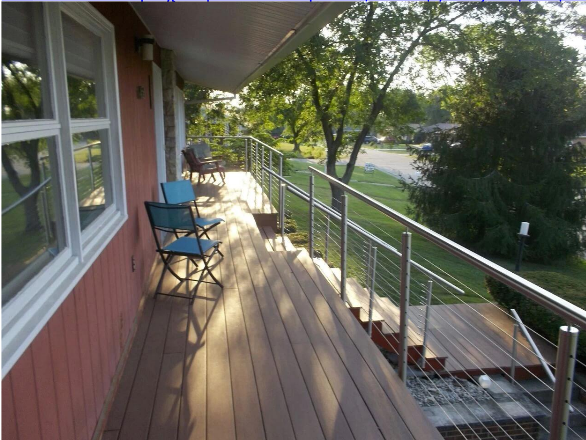
3. Stainless πλευρά γάλυβα mount κικκλίδωμα θέση για εξωτερικό μπαλκόνι :
