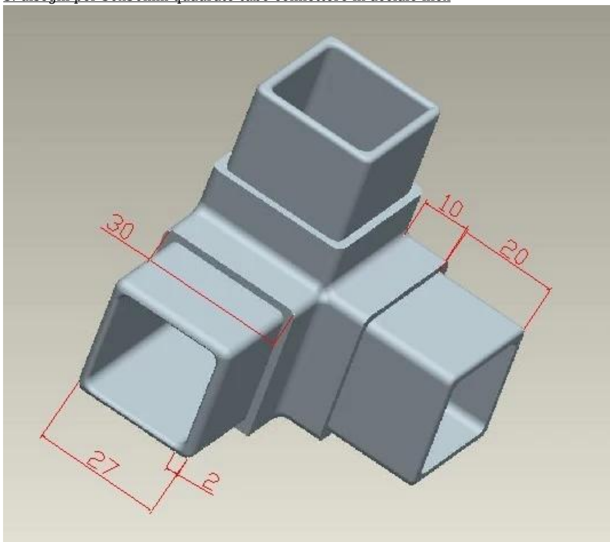
3. disegni per 30x30mm quadrato tubo connettore in acciaio inox
