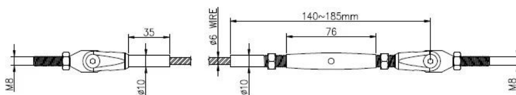
2) Wymiar napinacza linki T804
