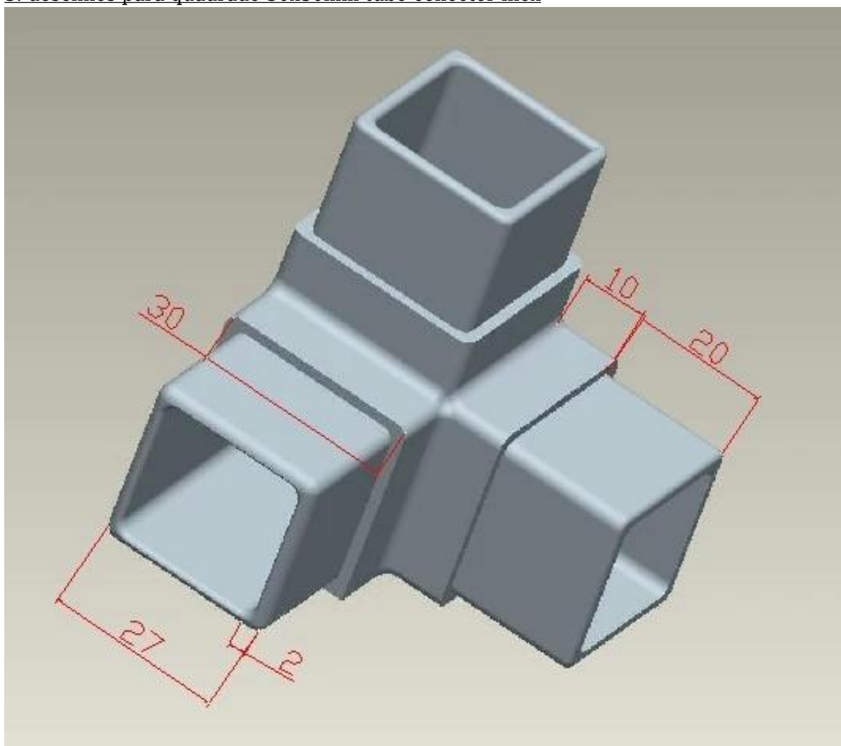
3. desenhos para quadrado 30x30mm tubo conector inox
