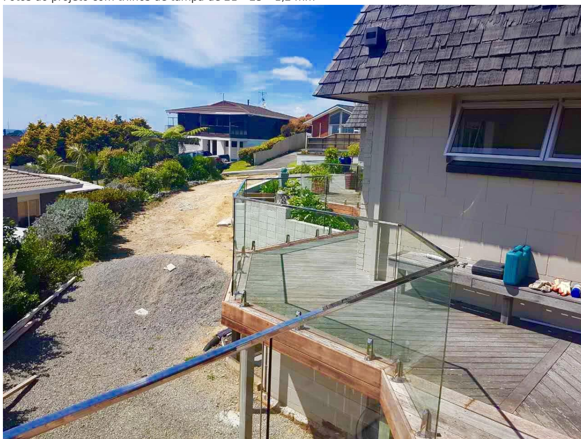
Fotos do projeto com trilhos de tampa de 21 * 25 * 1,2 mm-
