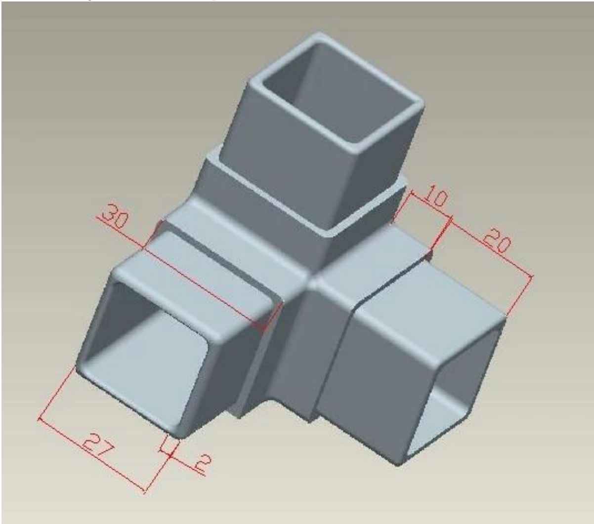
(3) Zeichnungen für 30x30mm quadratischen Rohr Verbinder Edelstahl
