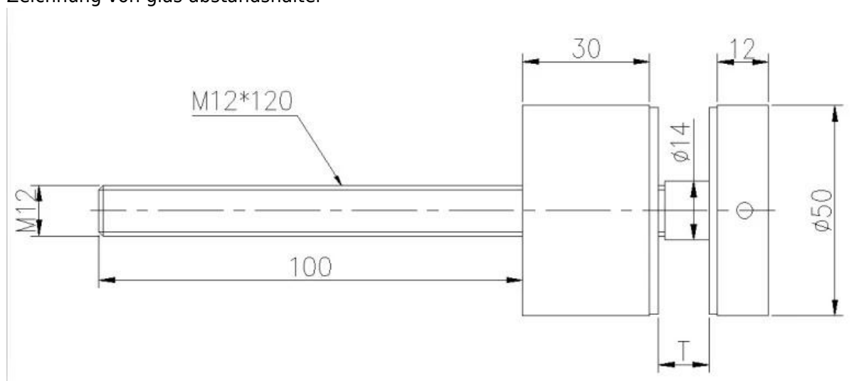
Zeichnung von glas abstandshalter
