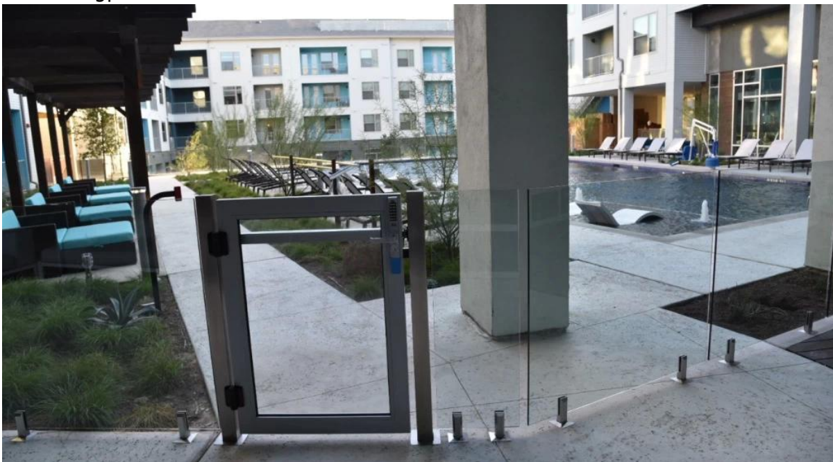
80x80mm Quadratpfosten und Glas verriegeln , Scharnier Entwurf für sicheres Swimmingpoolzauntor
