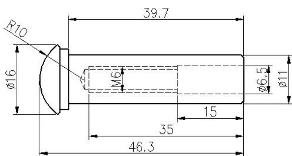
Zeichnung für Kabelgeländerspanner T807A-
