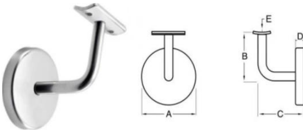
An der Wand befestigte Handlaufklammer technical Zeichnung
