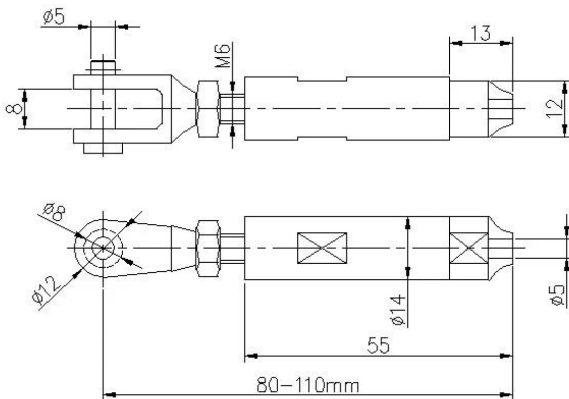
T803 Zeichnung
