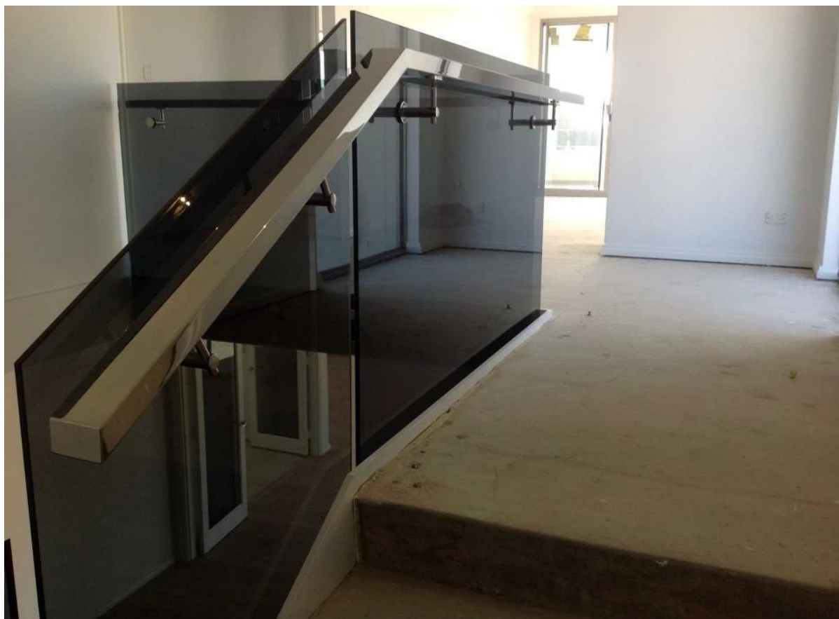
Barandilla de vidrio templado de 12mm con pasamanos de acero inoxidable
