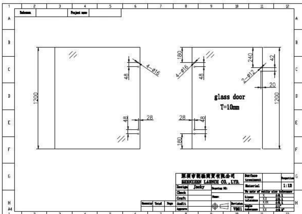
bisagra de puerta de vidrio orificios de panel de vidrio estándar posición de dibujo
