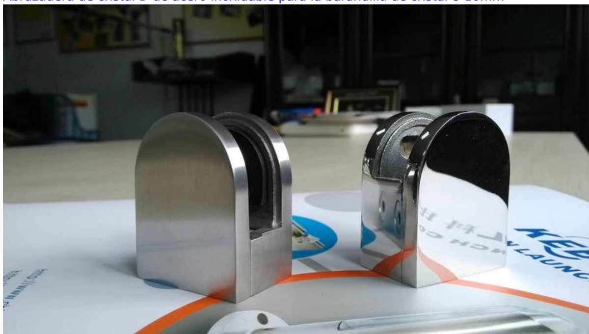
Abrazadera de cristal D de acero inoxidable para la barandilla de cristal 8-10mm
