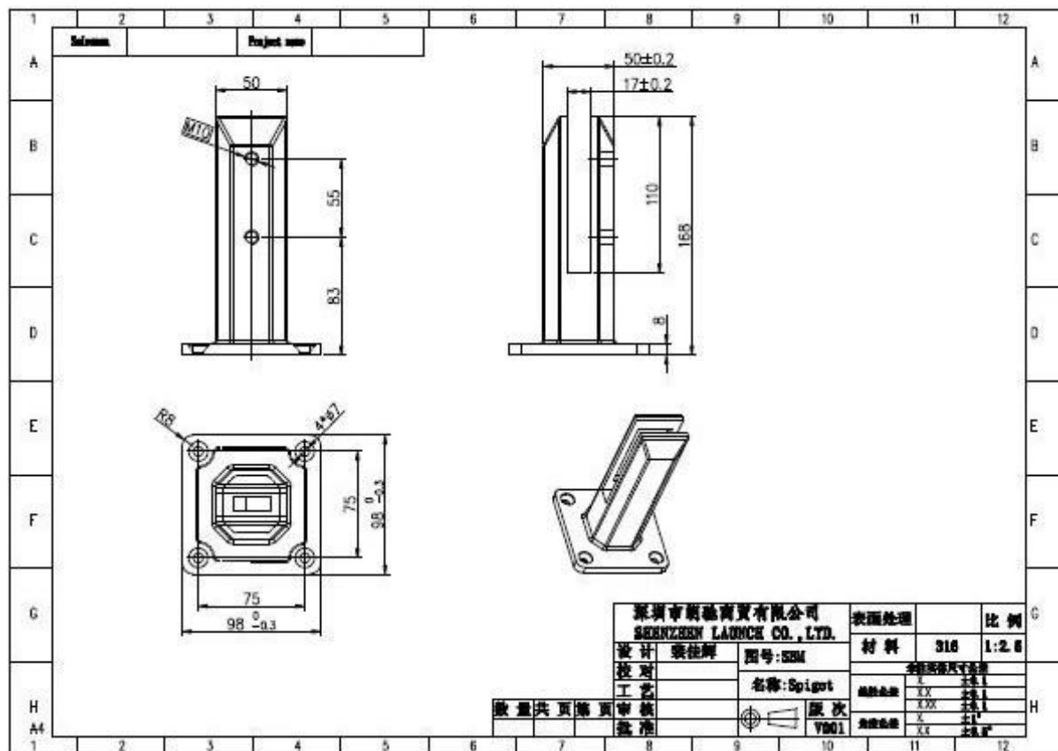
2. barandilla de vidrio sin marco acero inoxidable espiga fotos,
