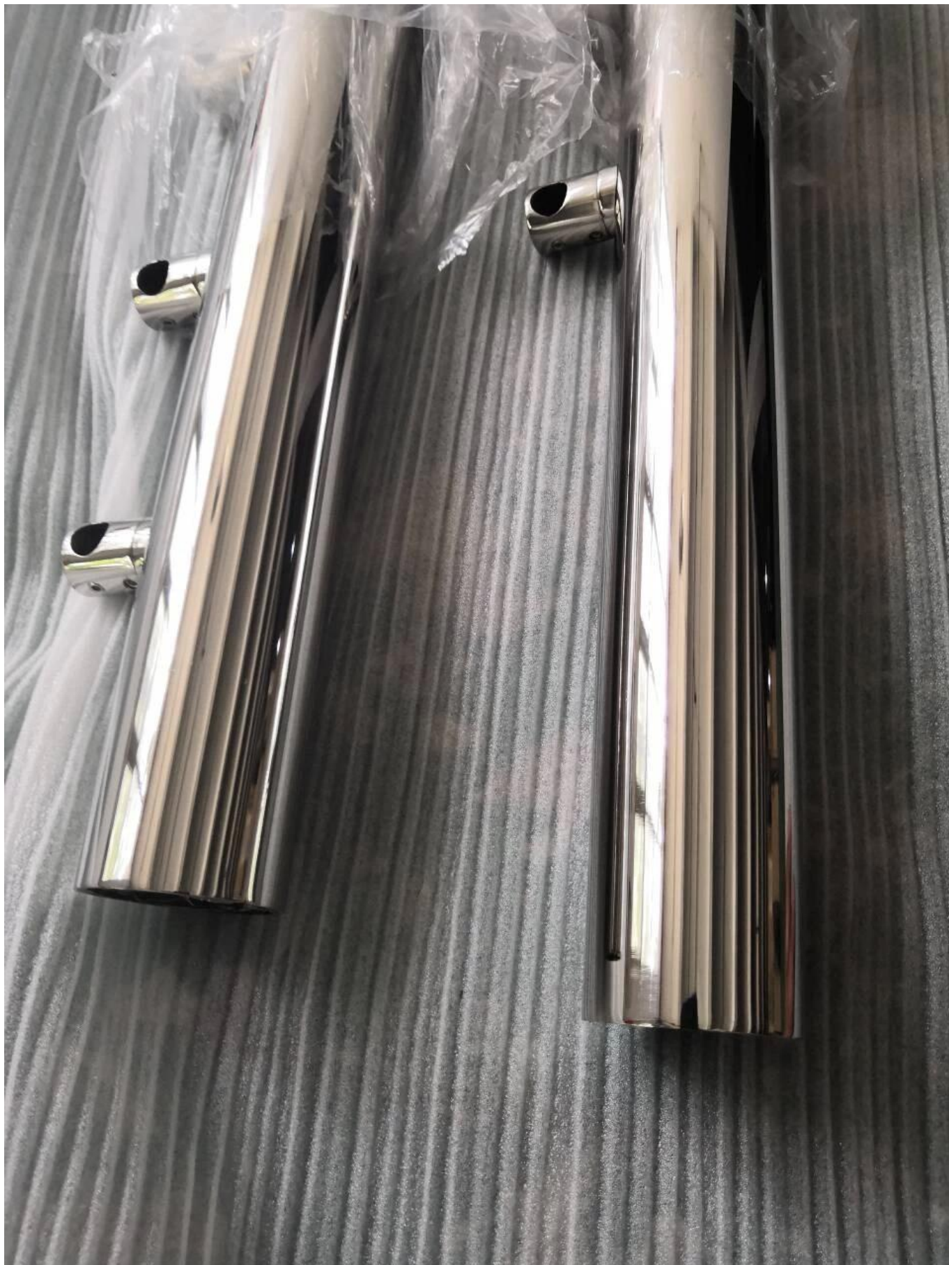
Vista superior de la barandilla de la barra transversal de acero inoxidable 316, con soportes de pasamanos ajustables
