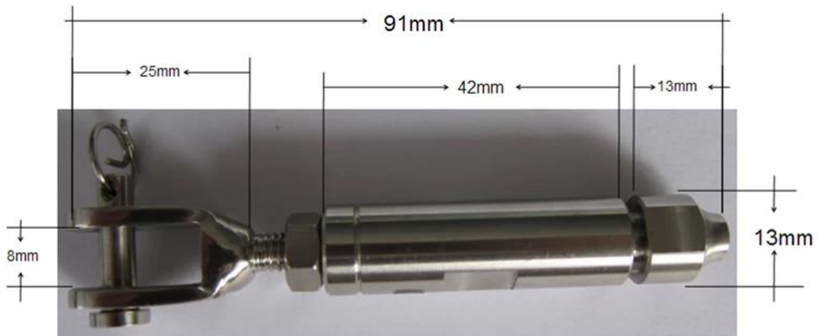
2) Kaapelin kiinnitys T803-mitta
