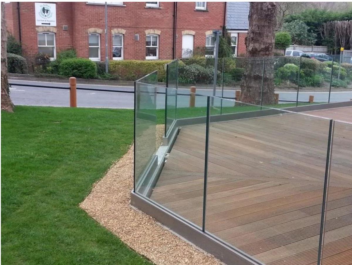
Alumiini U kanava + 10-12mm karkaistu lasi rakenne
