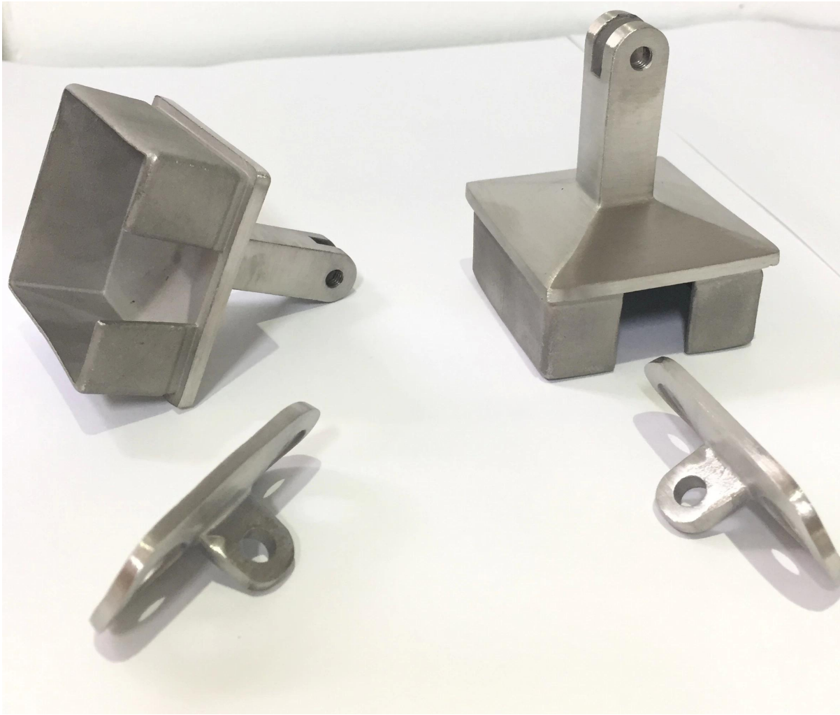
# Piirustus Uusi muotoilu 40x40mm säädettävä neliömäinen kaiteen kiinnike (malli NCF-40X)
