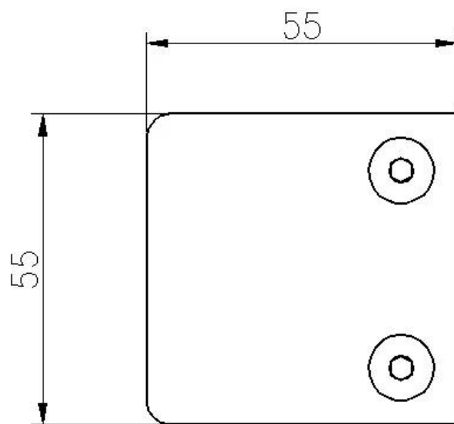
Lasipuristimen ulottuvuus
