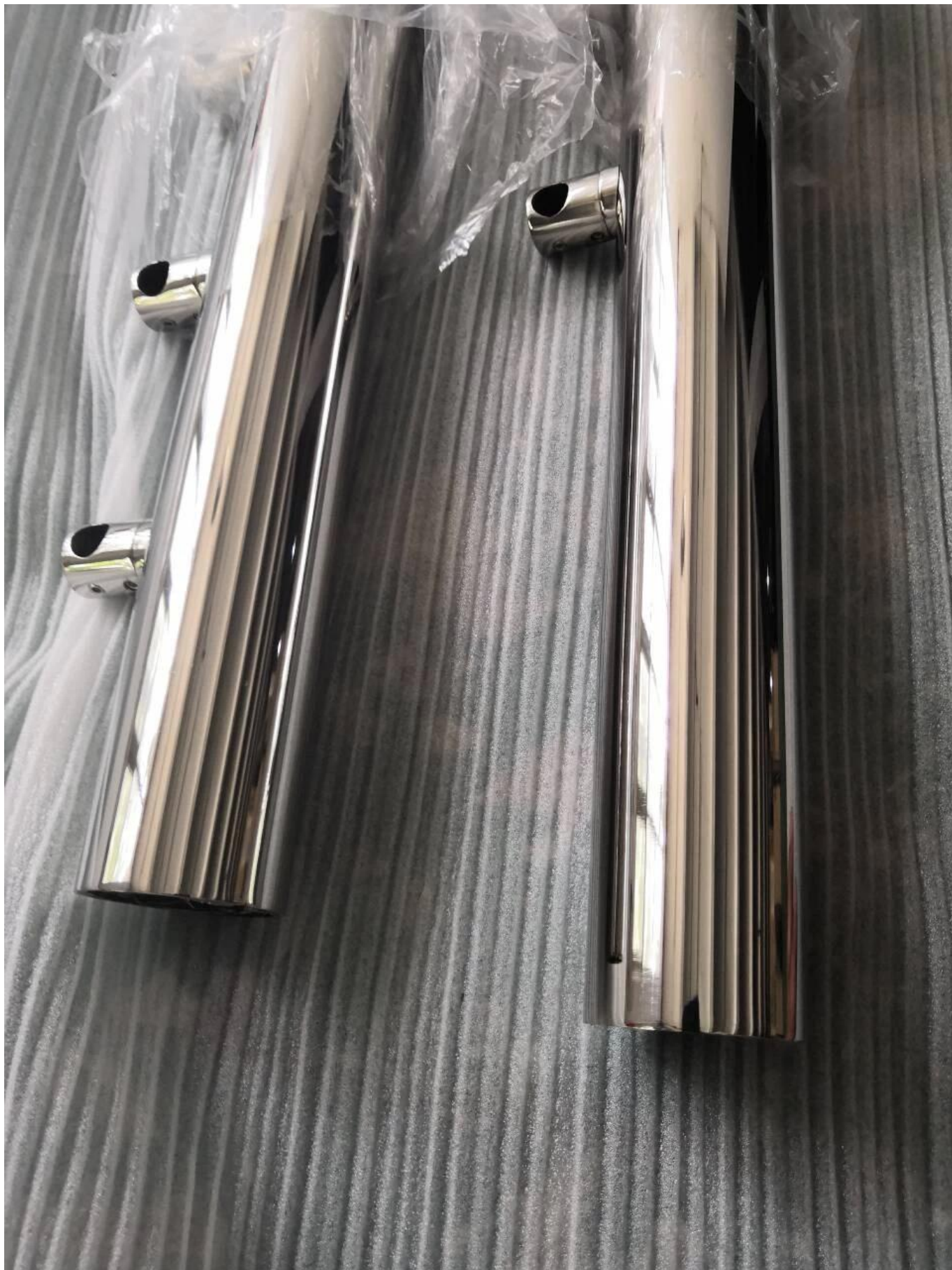
Ruostumattomasta teräksestä valmistettu 316 ruostumattomasta teräksestä valmistettu kaidepylväs ylhäältäpäin, säädettävillä kaidekiinnikkeillä
