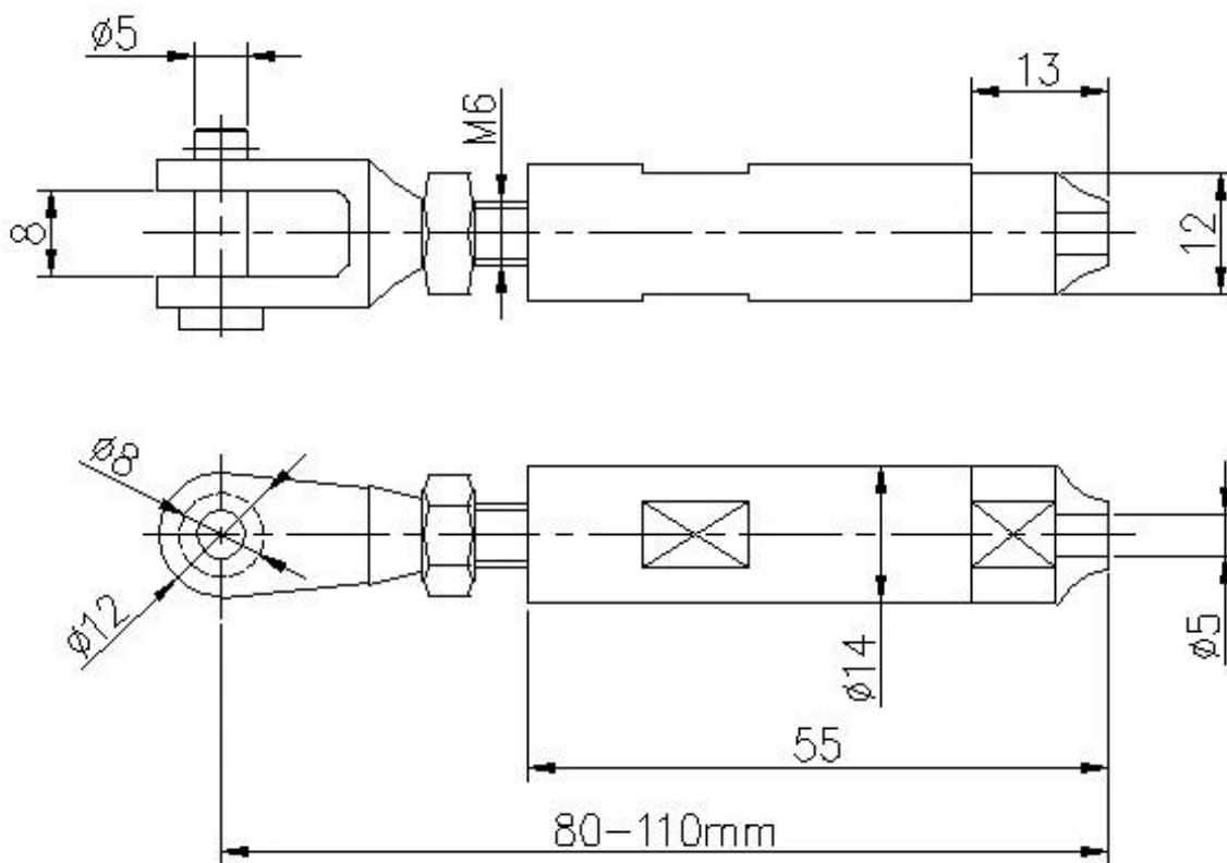
Piirustus kaapelikiskojen laitteistosta T803
