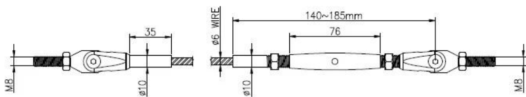
2) Dimension du tendeur de câble T804
