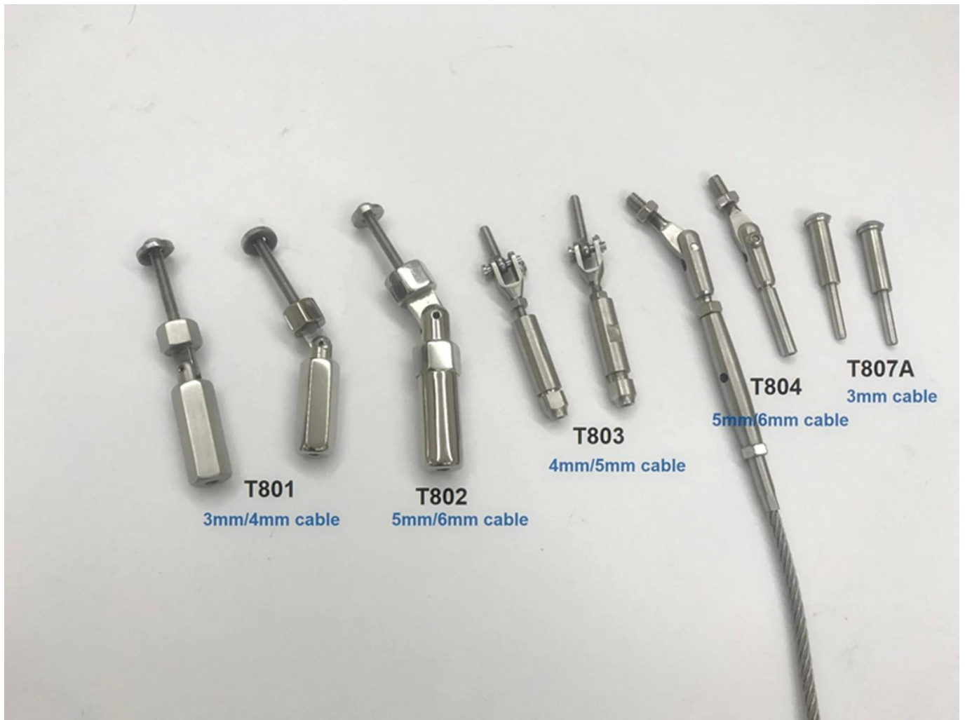
Designs de garde-corps de câbles avec tendeurs -
