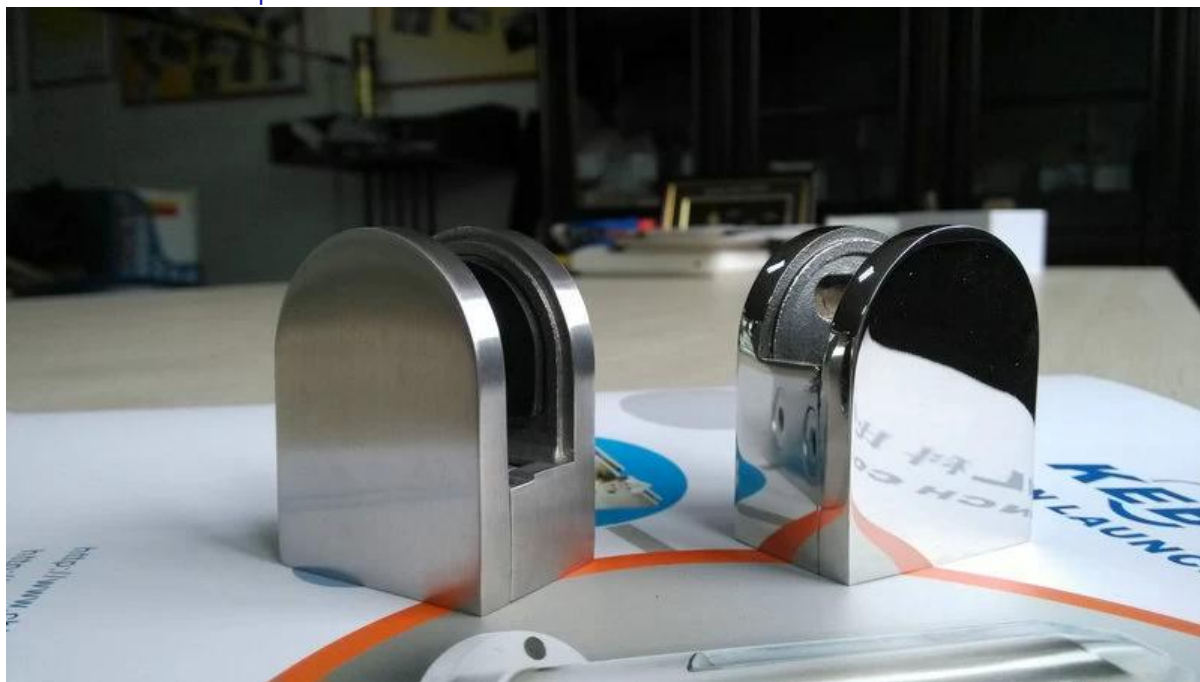
Collier inox verre D pour 8-10mm balustrade en verre
