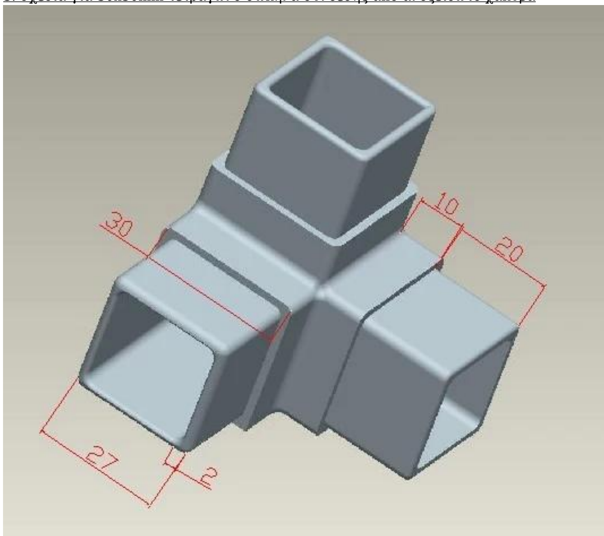
3. σχέδια για 30x30mm τετράγωνο σωλήνα σύνδεσης από ανοξείδωτο χάλυβα
