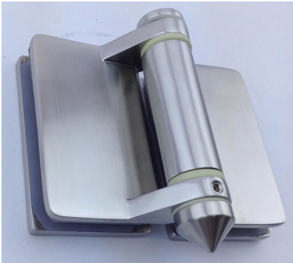
Γυαλί στο στρογγυλό μεντεσέ (στρογγυλή διάμετρος στηρίγματος 50,8 mm)
