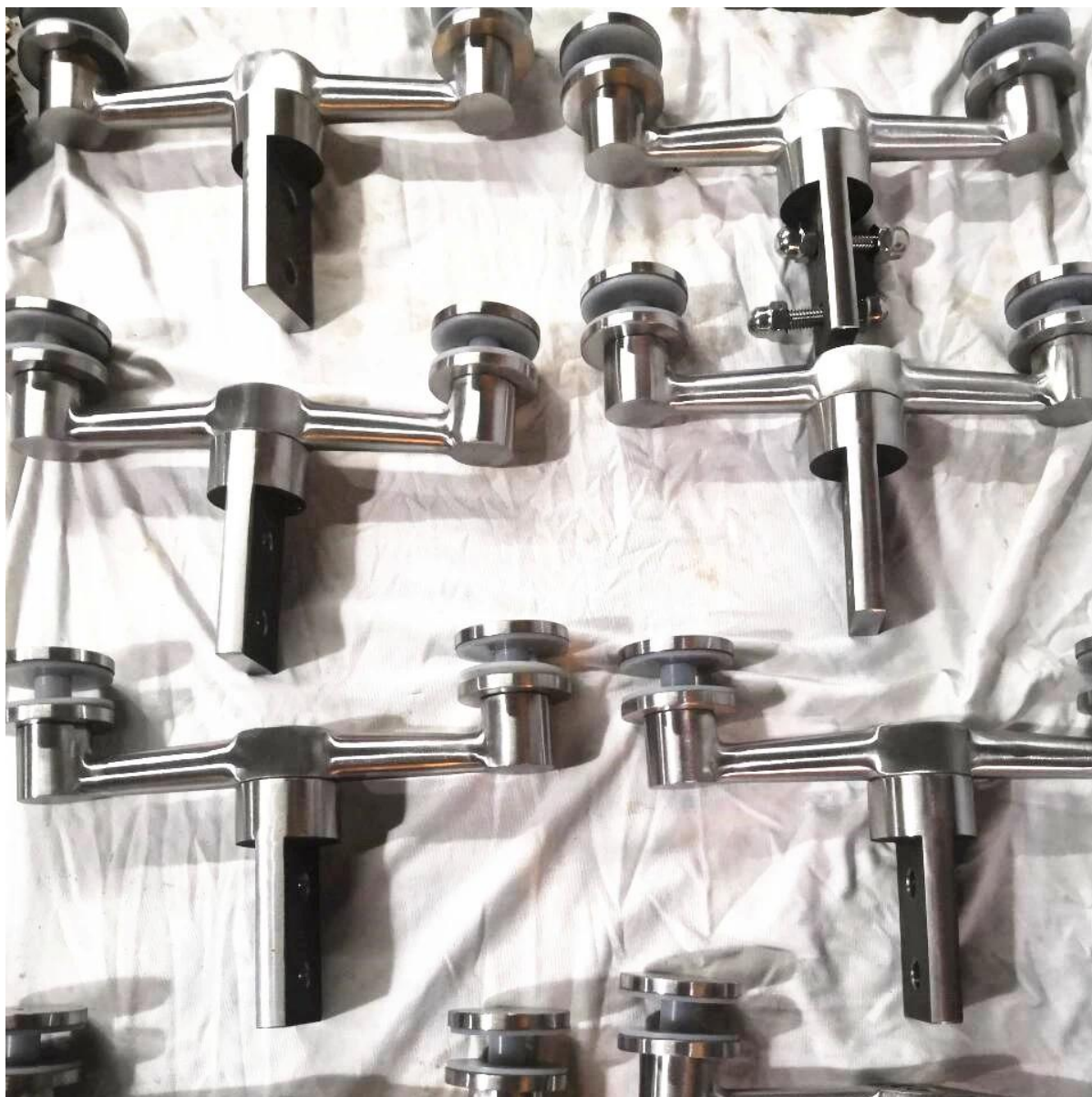
Φωτογραφία του έργου της τοποθέτησης υαλοπίνακα για τοίχους κουρτινών -
