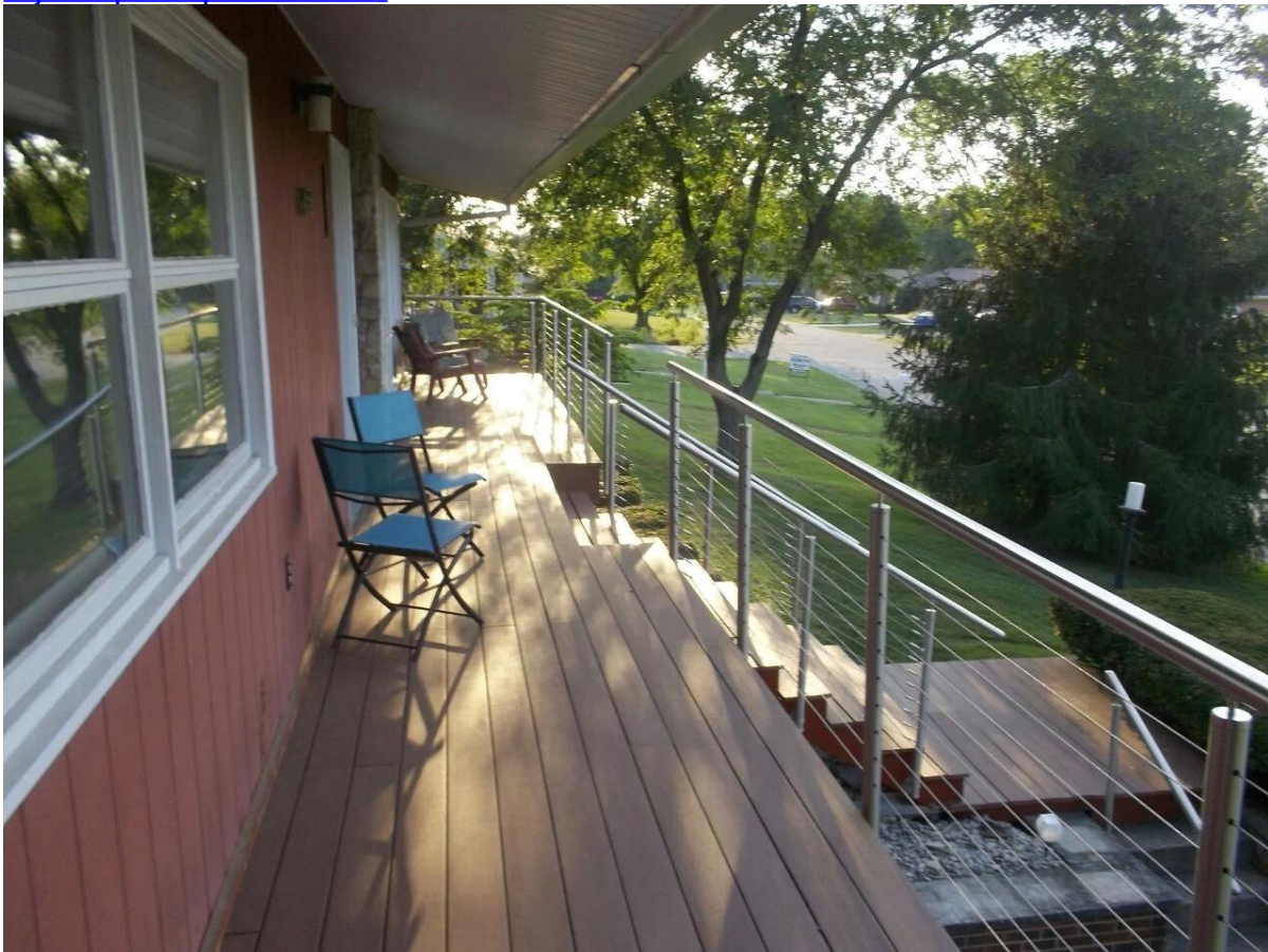
3. Side mount ανοξείδωτο χάλυβα σχεδιασμό καλώδιο κιγκλίδωμα για εξωτερικό μπαλκόνι :
