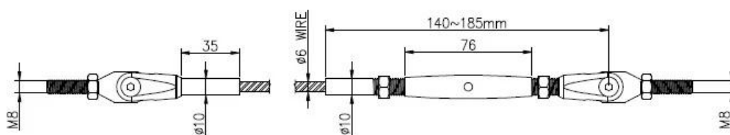
2) Dimensioni del cavo T804
