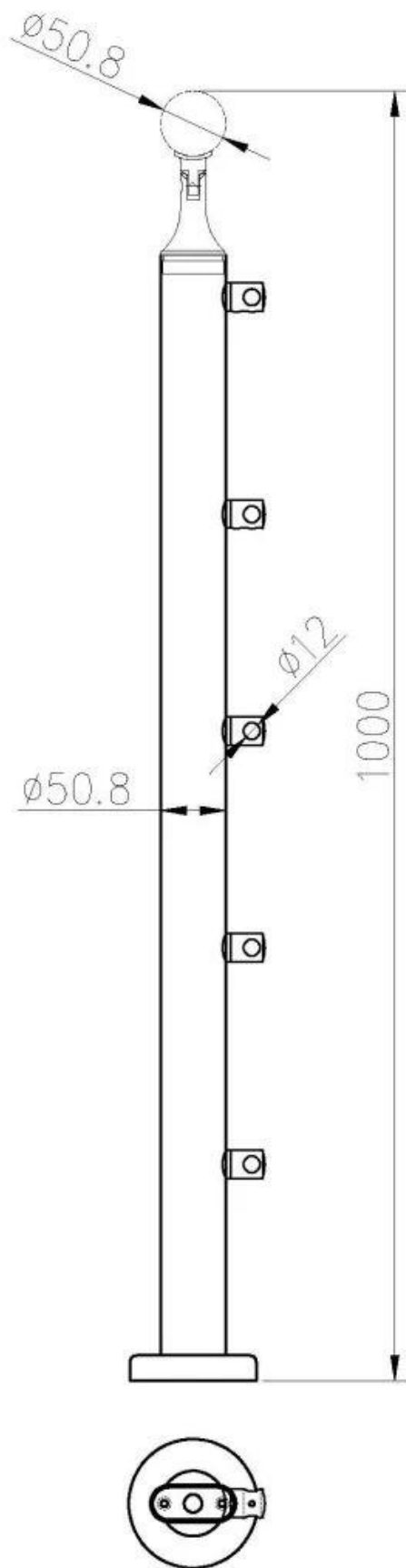
Disegno di progetto della scala a chiocciola
