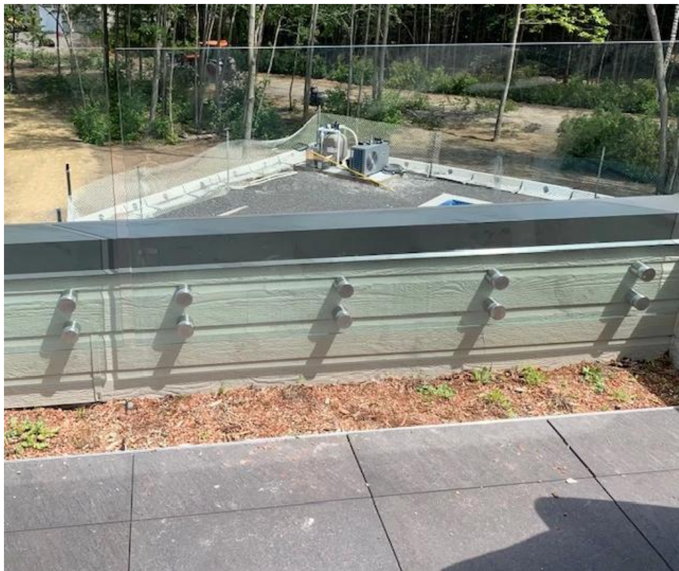
Standard in vetro in acciaio inox per balaustra in vetro senza telaio
