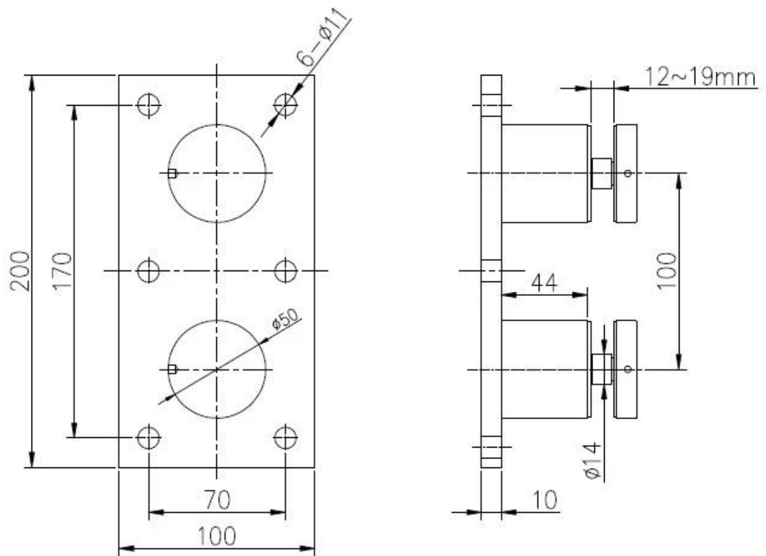
Disegno tecnico:
