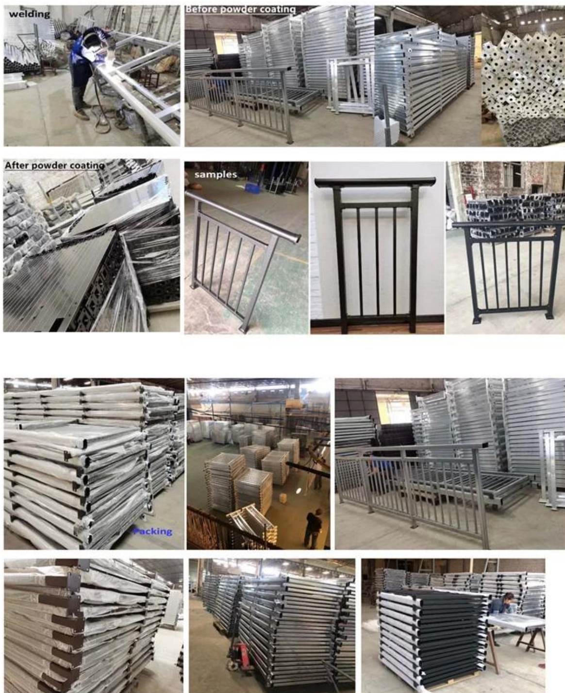
Foto del progetto della recinzione in acciaio zincato
