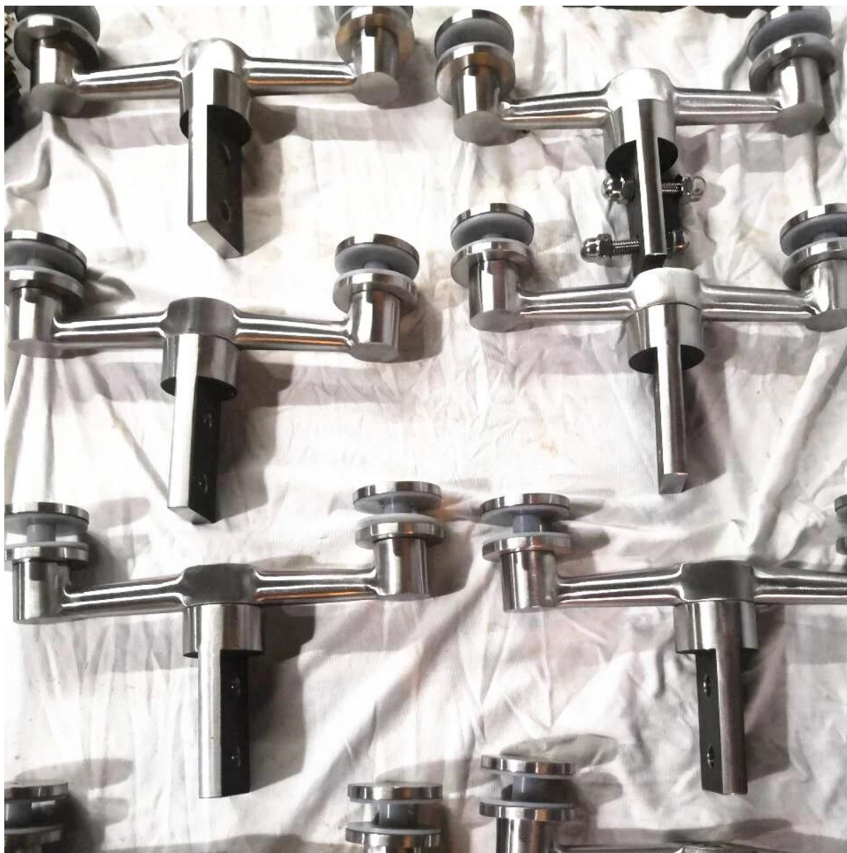
Foto di progetto di montatura in vetro ragno per facciate continue -
