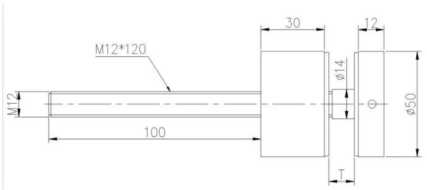
staffa di supporto in vetro in acciaio inossidabile
