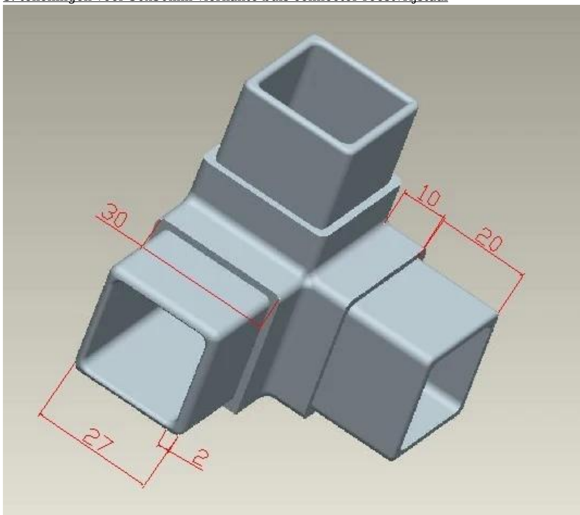
3. tekeningen voor 30x30mm vierkante buis connector roestvrijstaal
