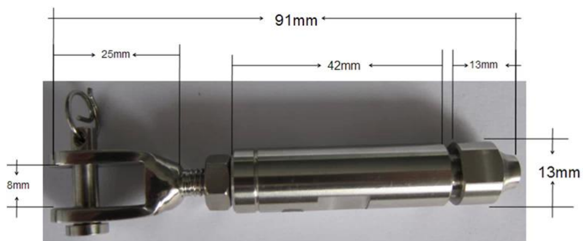
2) T803-afmeting van de kabelrailing
