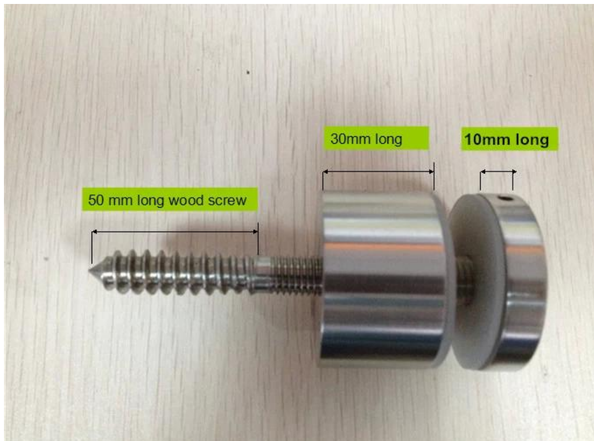
Afmetingen van glas impasse pin.
