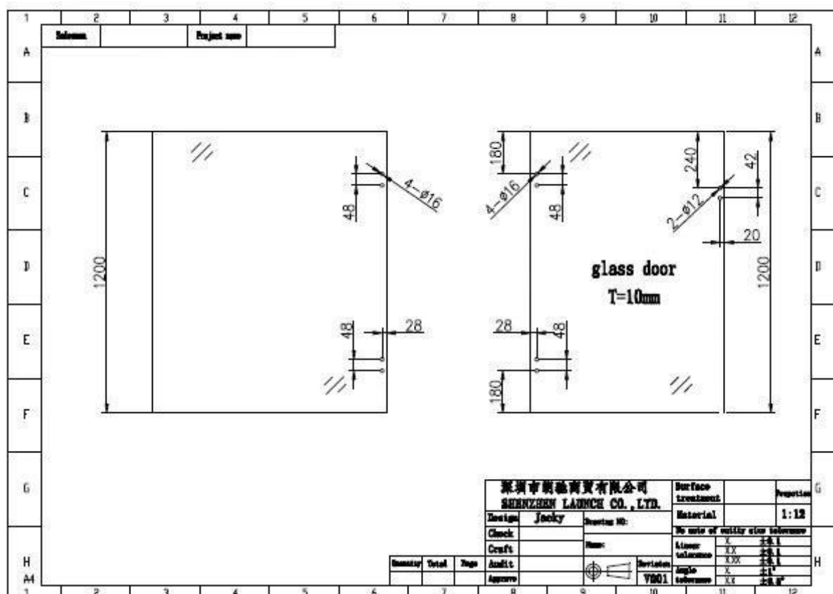
glazen deurscharnier standaard glaspanelen positiepositie tekening
