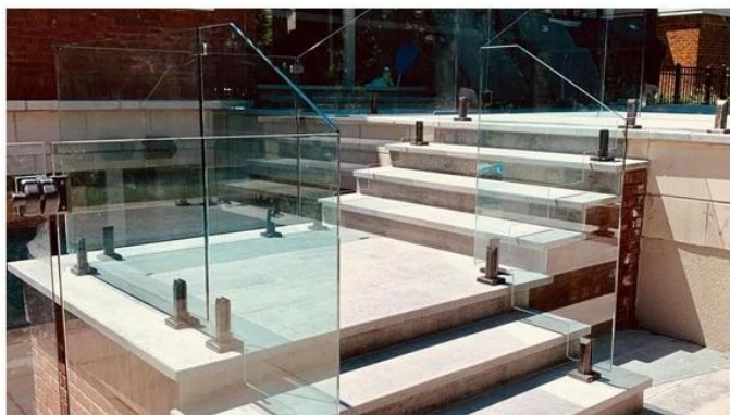
Satijn geborsteld Roestvrijstalen hekklem Glas zwembad hek Spigot SBM-3:
