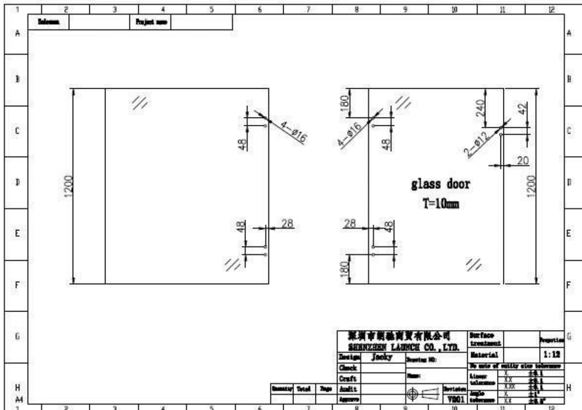
glazen deur scharnier standaard glazen paneel gaten positie tekening
