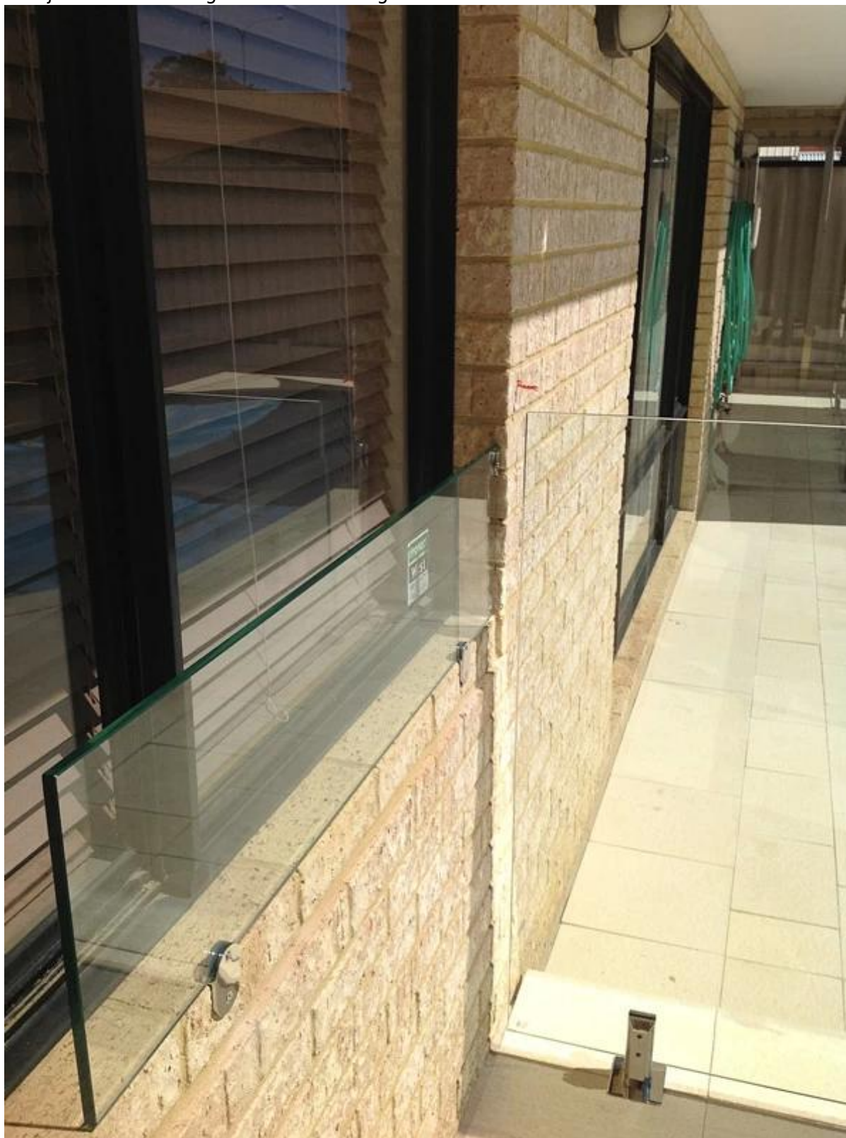
- Projectfoto van een glasklem van 180 graden naar muur
