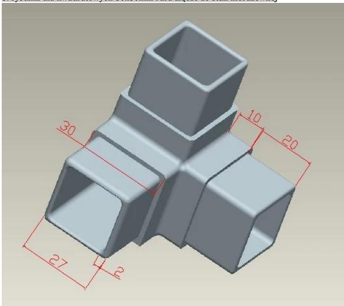
3. rysunki dla kwadratowych 30x30mm rura złącze ze stali nierdzewnej
