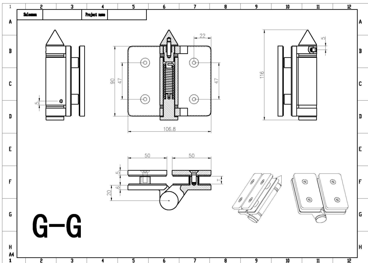
Rysunek do otworów do 316 stali nierdzewnej samozamykające szklane bramy basenowe -
