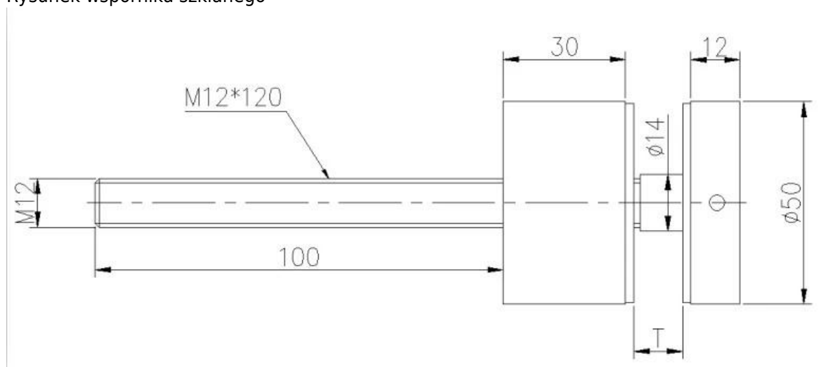
Rysunek wspornika szklanego
