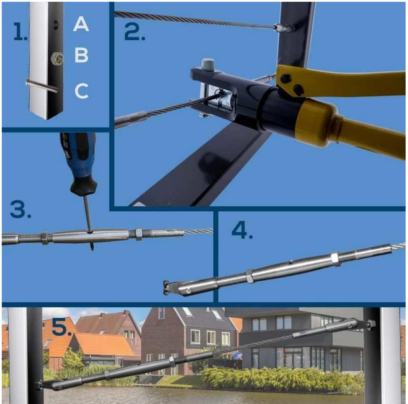
Zdjęcie balustrady kablowej Zdjęcie:
